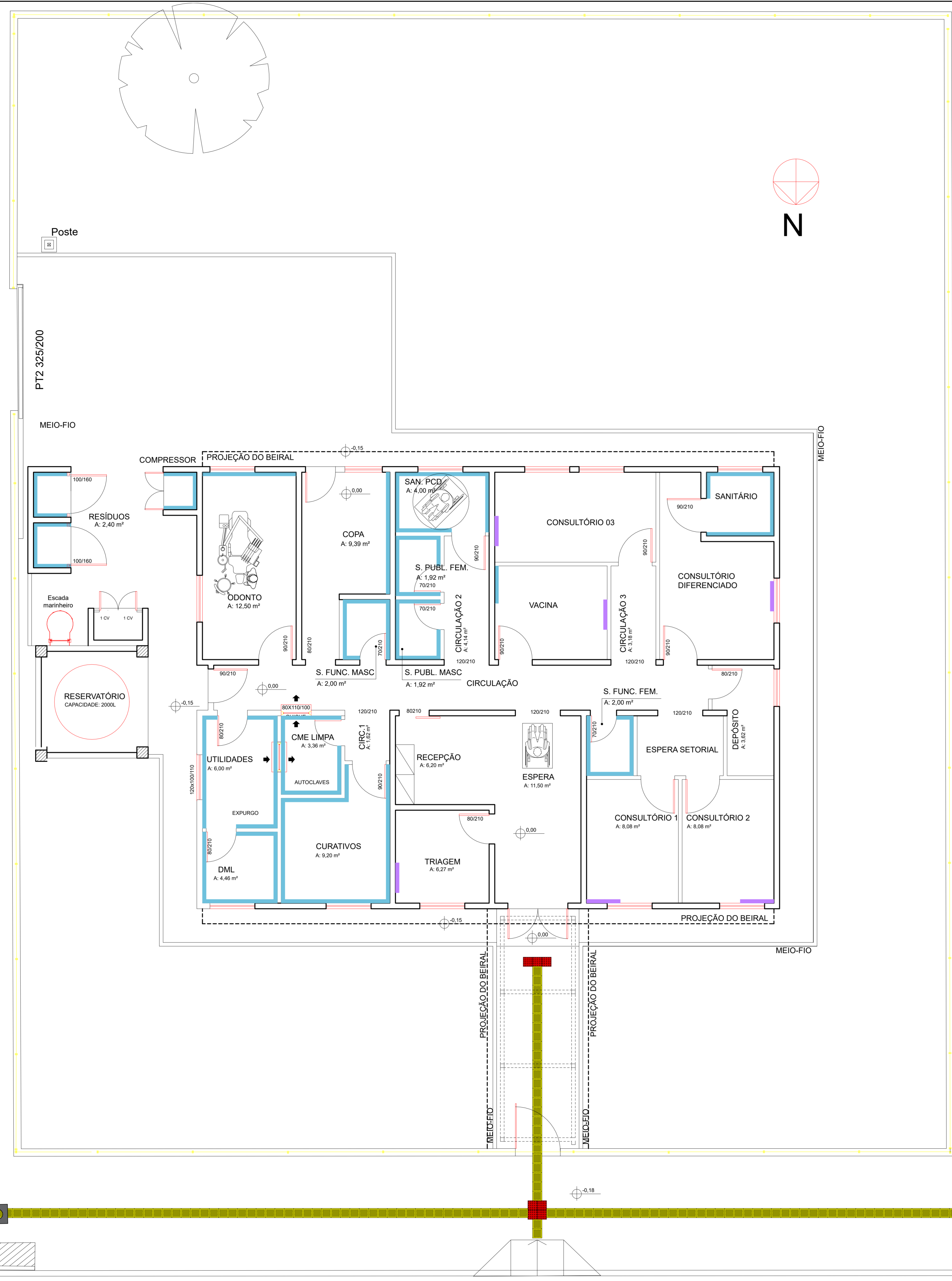
PLANTA LAYOUT ESCALA: 1/50 A= 183.49 m2
