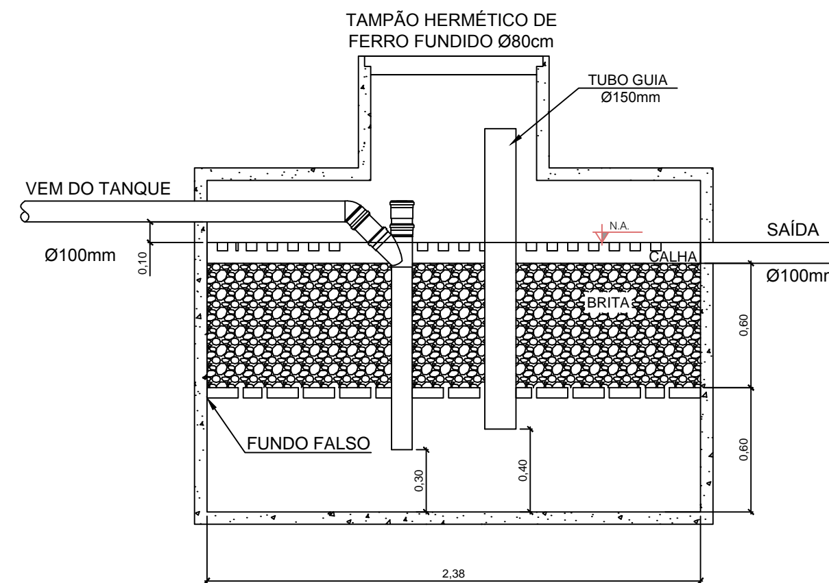
CORTE
