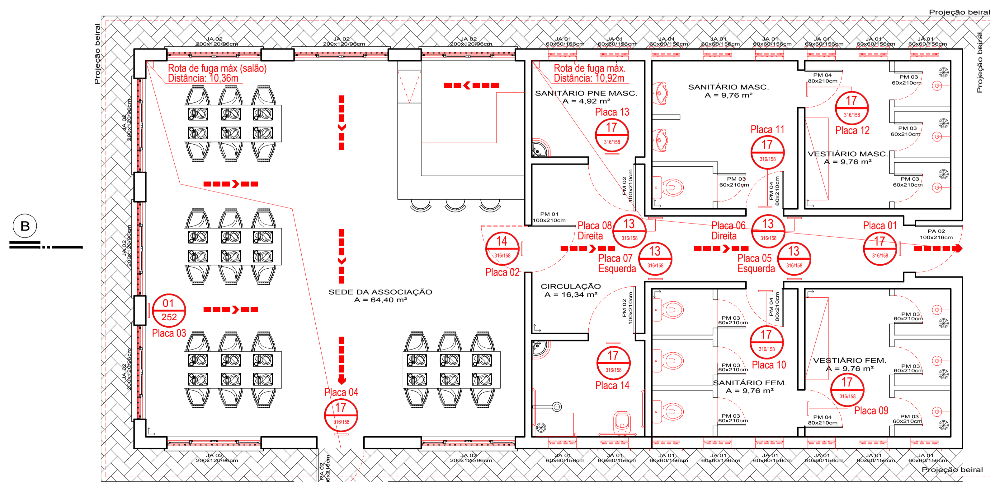
PLANTA BAIXA - SINALIZAÇÃO/ROTAS DE FUGA ESC. 1:50
