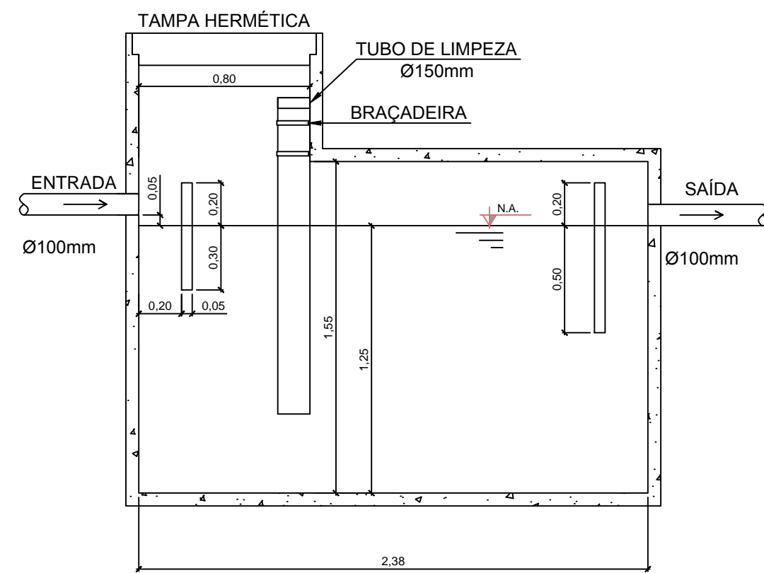
CORTE
