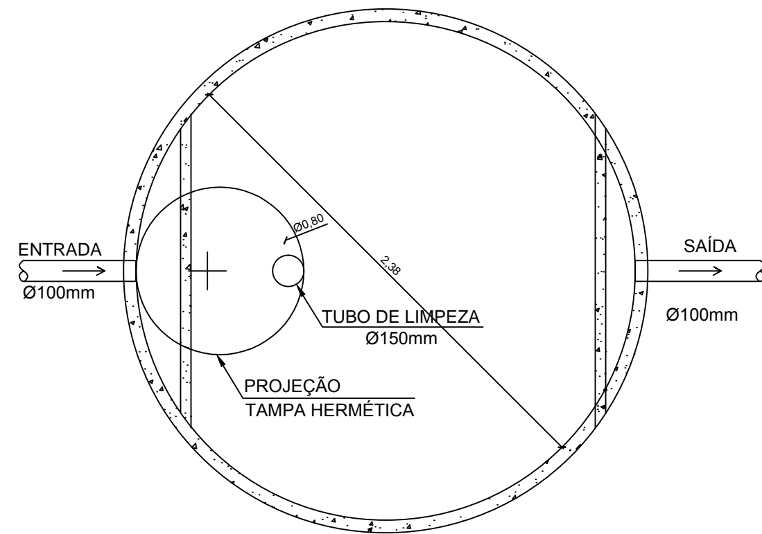
PLANTA
