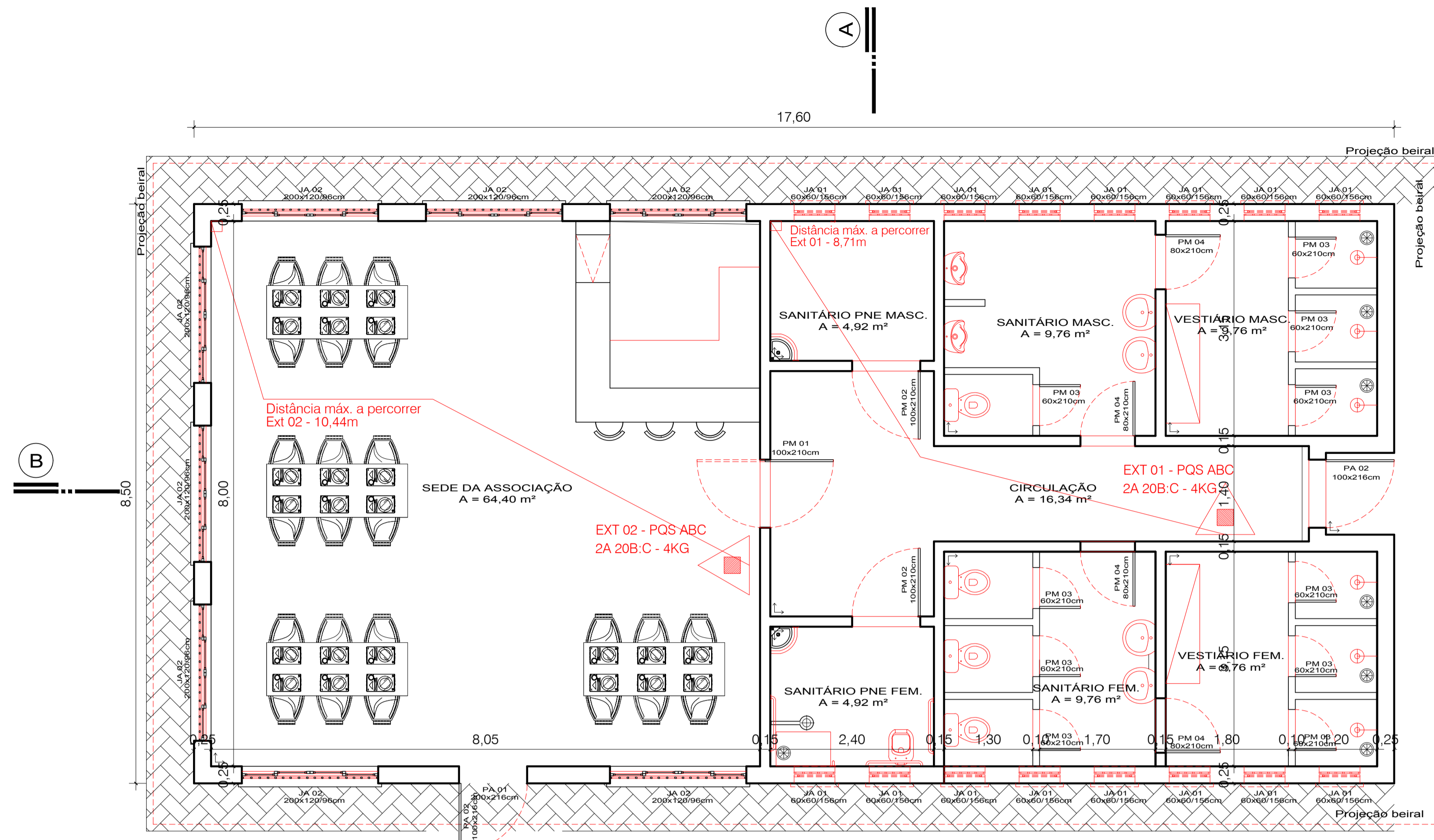
PLANTA BAIXA - EXTINTORES DE INCÊNDIO ESC. 1:50
